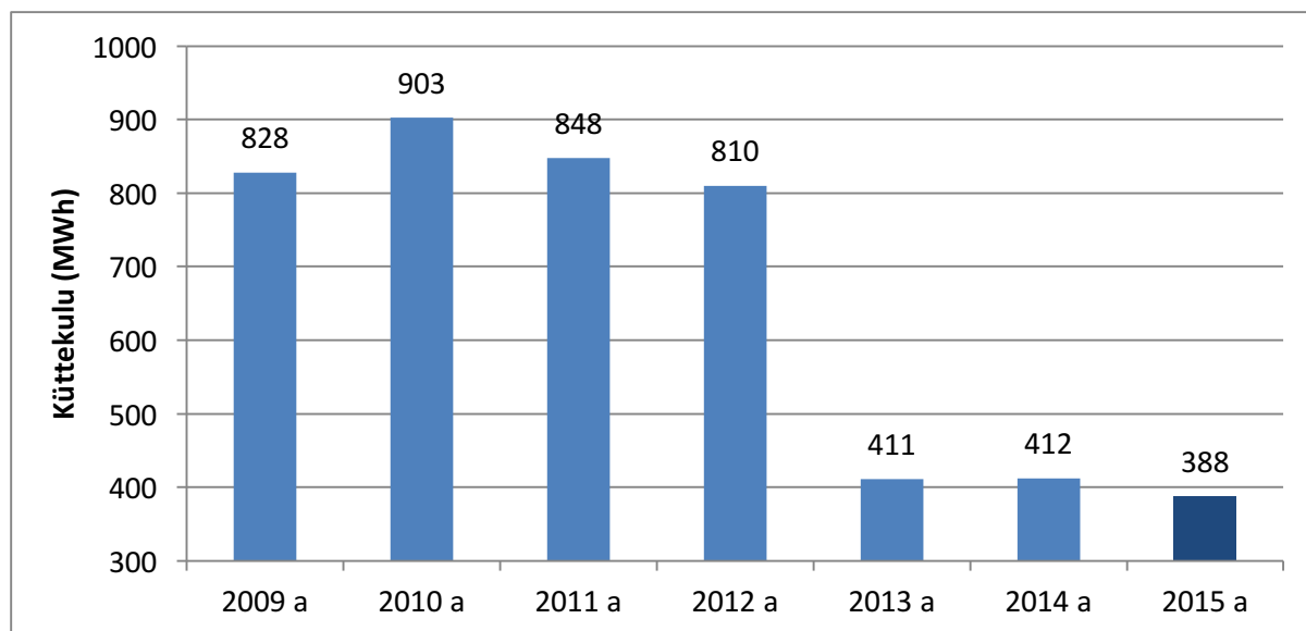
Joonis 1. SA Haapsalu Neuroloogilise Rehabilitatsioonikeskus kütteenergia tarbimine haiglahoones renoveeritud 5367 m 2 kohta 2009. – 2015. aastal.
